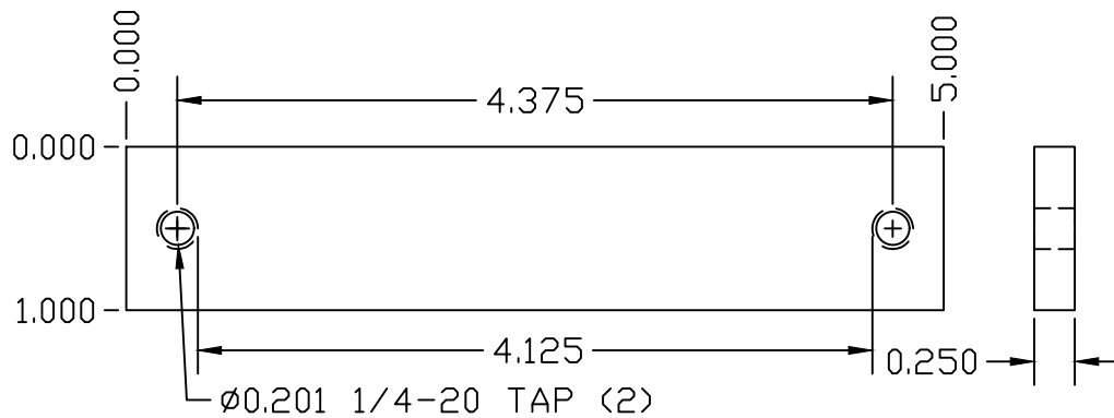
BOTTOM CLAMP
